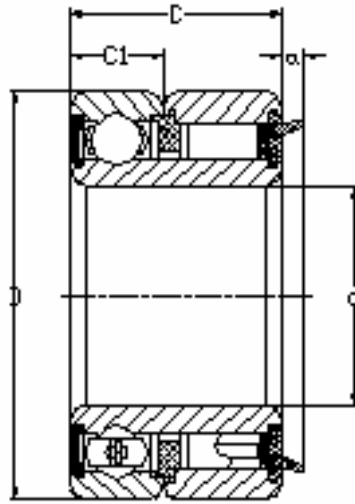
圆柱滚子离合器和球轴承组件
